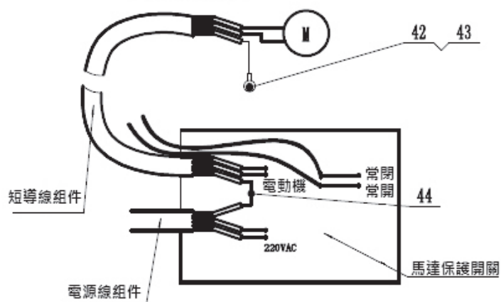
接線原理圖
